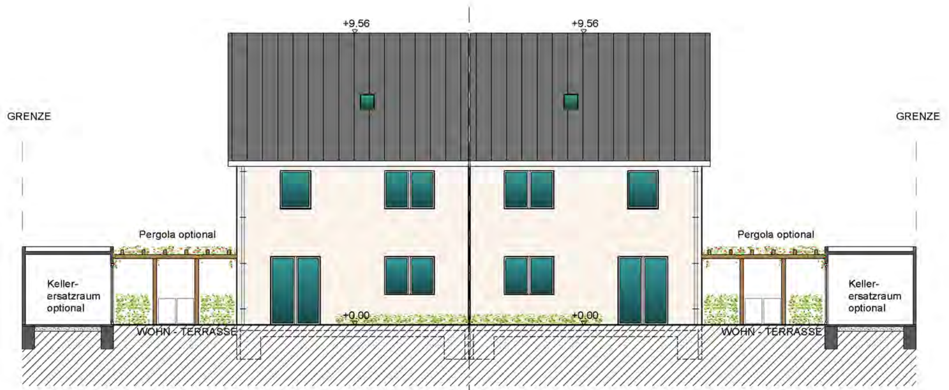
ANSICHT NORD oder SÜD
